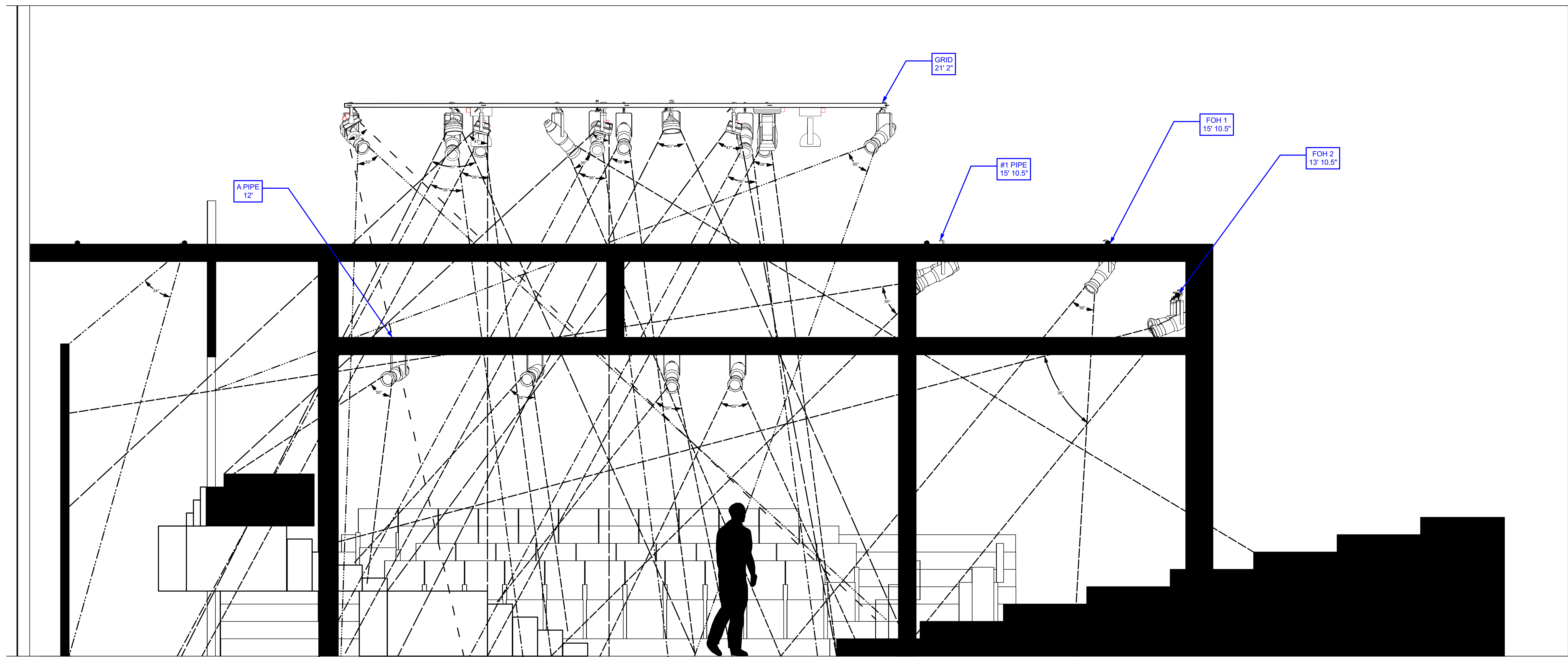
1 Section Scale: 1/2" = 1'-0"
